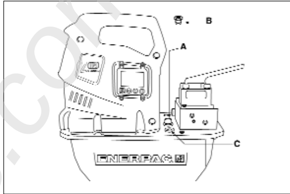
Kuva 2, ZU4-tuuletusaukon asennus
