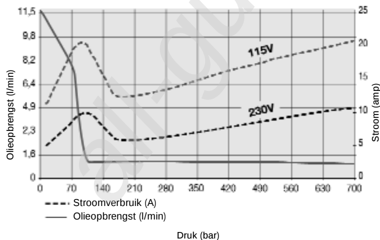
Olieopbrengst en stroomverbruik vs. druk
