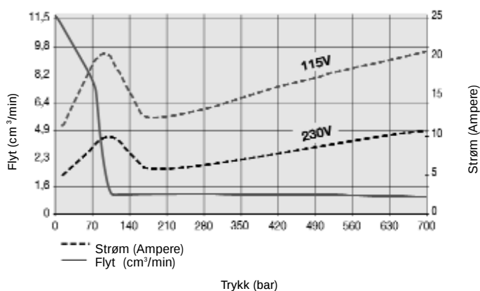
Flyt og Elektrisitet vs. Trykk
