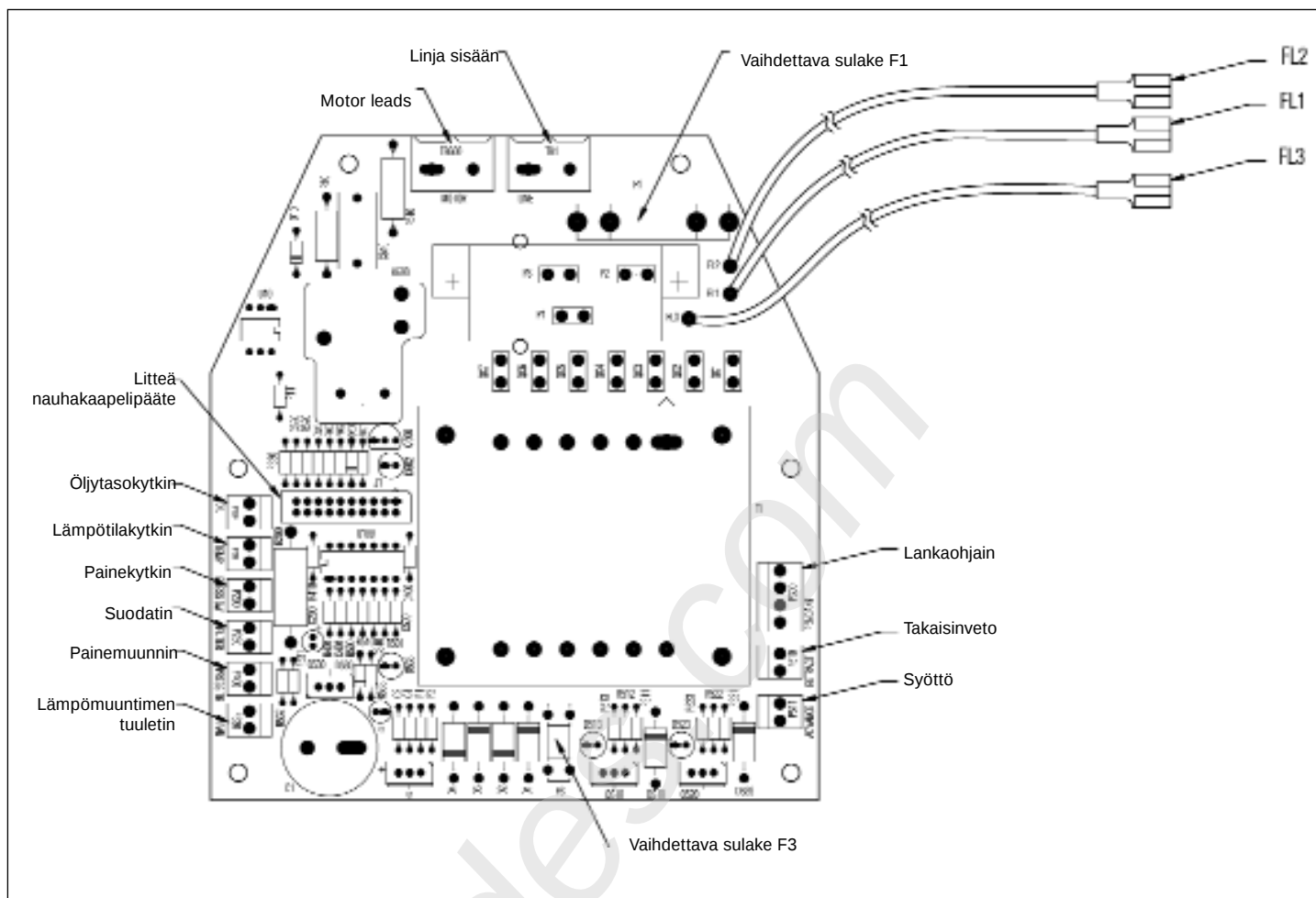
Kuva 12, sähkövirtapaneelin kokoonpano
